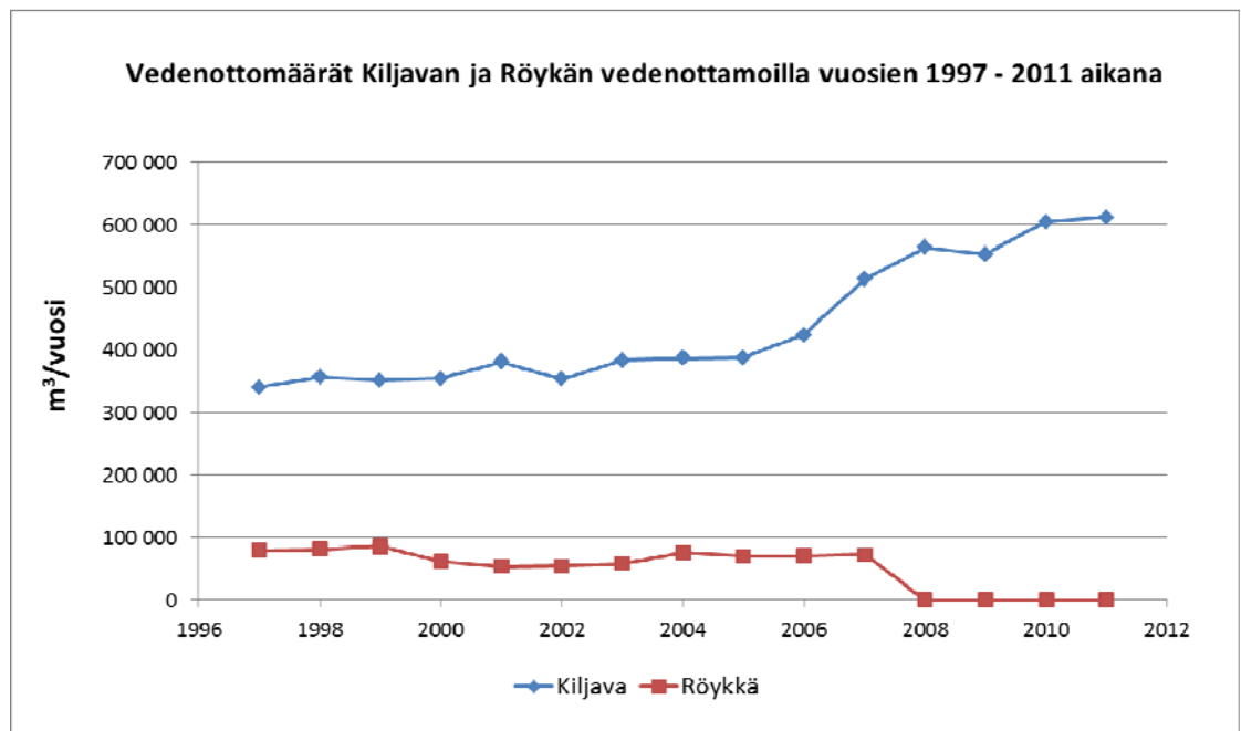
Kuva 4. Kiljavan ja Röykän vedenottamoiden vedenottomäärät vuosina 1997 - 2011.
